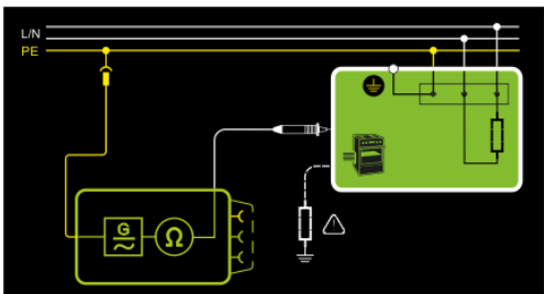
Hilfe – Prinzip- und Anschlussbild
