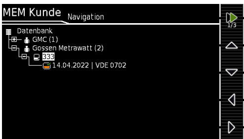
Datenbankstruktur – Kundenliste
