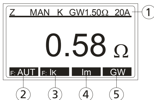
Bild 8: Messfunktion Zi
