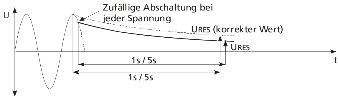
Bild 13: Linearer Modus
