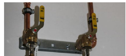
Belastungs- und Dichtheitsprüfung oder Leckmengenmessung mit Y-Verteiler zur gleichzeitigen Messung der Verteiler- und Verbrauchsleitung
