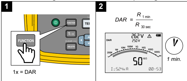
Abbildung 6. Dielektrischer Absorptionsgrad
