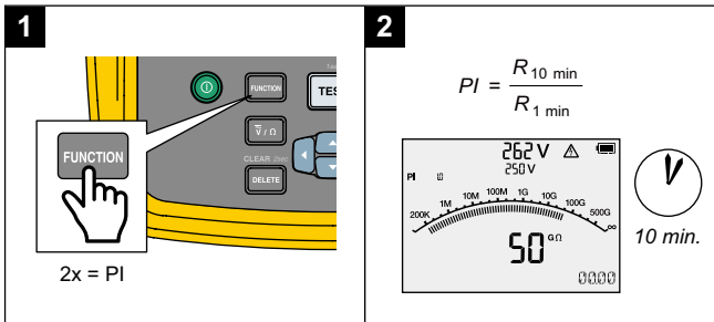
Abbildung 4. Polarisationsindex (PI)
