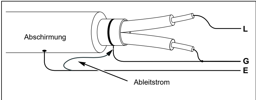
Abbildung 3: Verbesserte Guardanschluss-Verbindung
