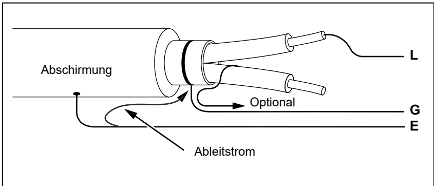
Abbildung 2: Guardanschluss-Verbindung
