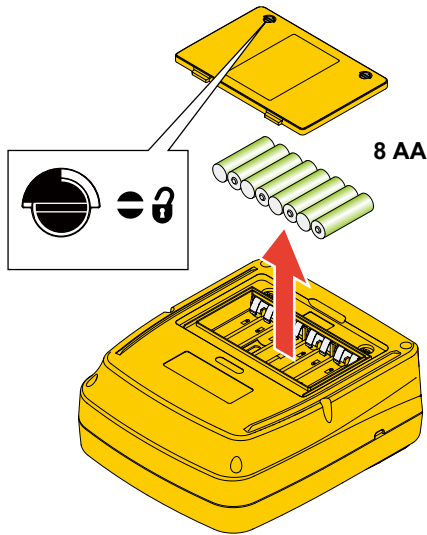
Abbildung 11. Austauschen der Batterien
