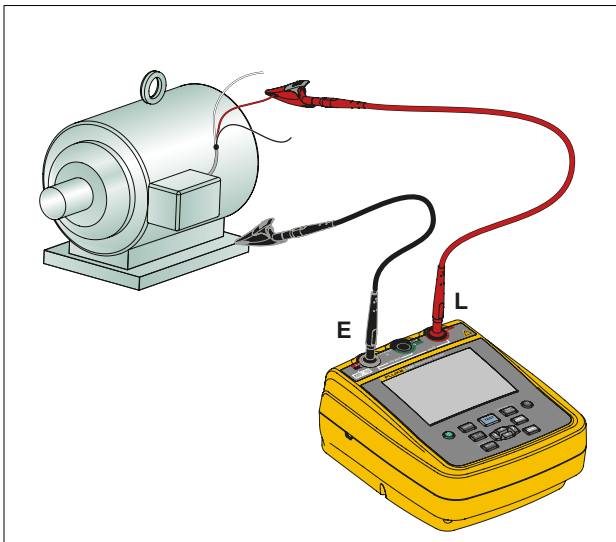
Abbildung 7. Verbindungen für Isolationsprüfung
