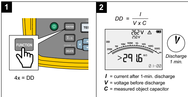
Abbildung 5. Dielektrische Entladung
