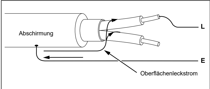
Abbildung 1. Ableitstrom
