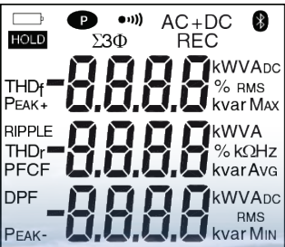
Anzeigefenster der Modelle F407 und F607
